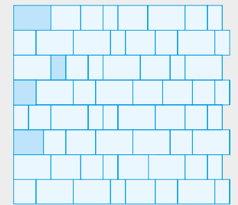
Gemischter Reihenverband mit 4 Formaten 26,25 x 17,5; 17,5 x 15,75; 21 x 17,5 und 17,5 x 10,5 cm
