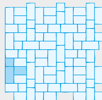
Wilder Verband mit 3 Formaten 12,6 x 12,6; 18,9 x 12,6; 25,2 x 12,6 cm
