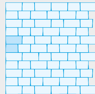
Reihenverband mit 2 Formaten 18,9 x 12,6; 25,2 x 12,6 cm
