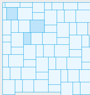
Wilder Verband "Muster 8" 17,5 x 10,5; 17,5 x 15,75 und 21 x 15,75 cm
