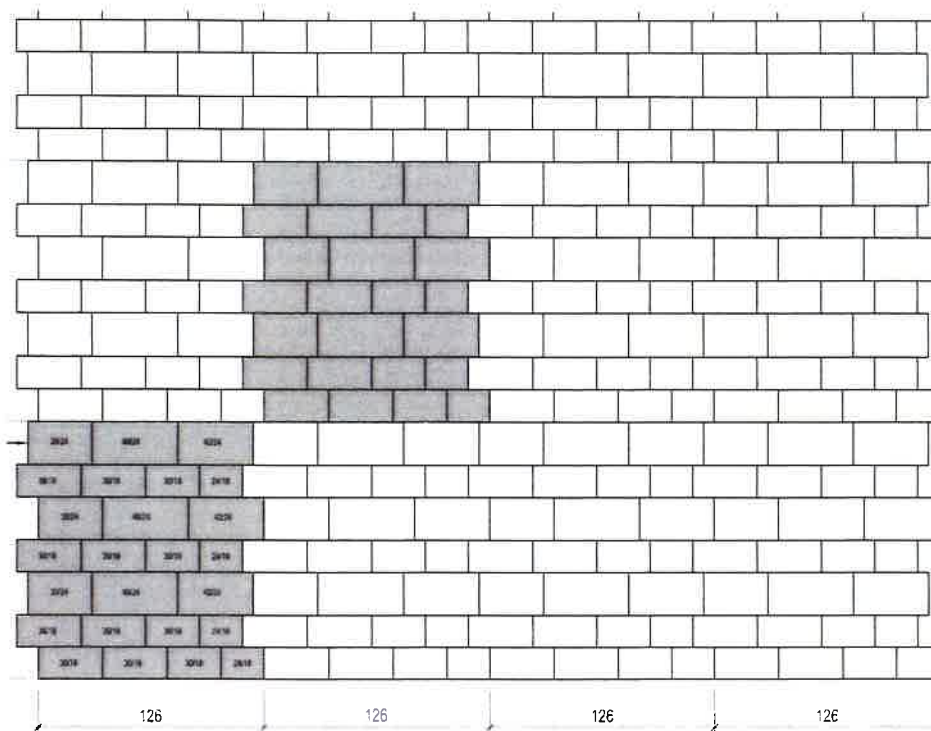
Bild: CityTruck 12 cm, Mixformen Typ D und E, Verlegebild
